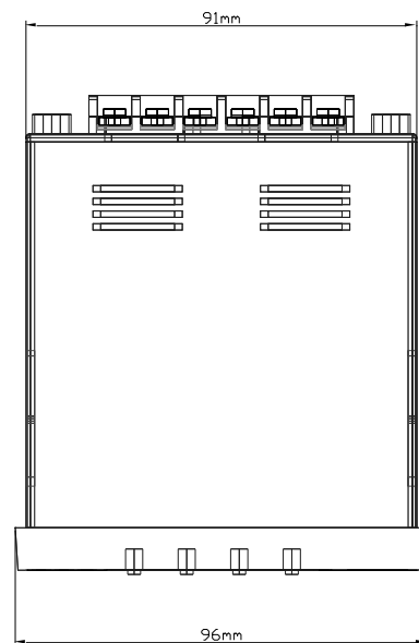
Fig. 5 – Vista superior
